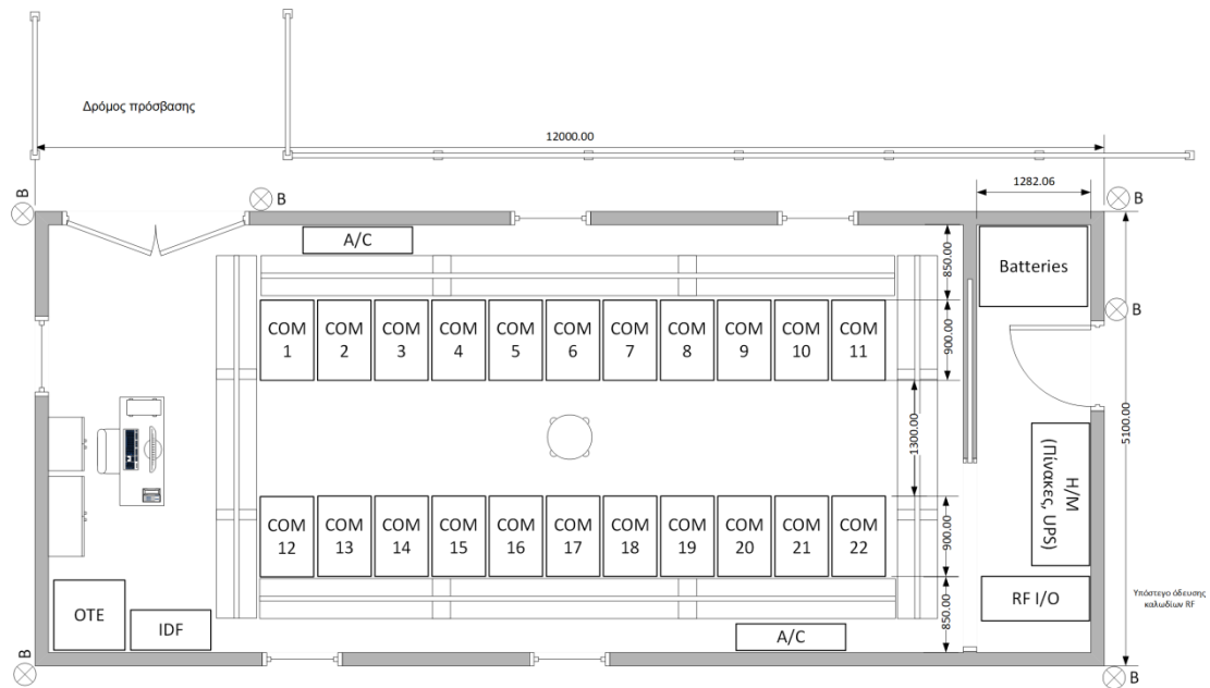
Σχέδιο 3: Διαρρύθμιση εσωτερικού χώρου νέου οικίσκου και θέση Η/Μ συστημάτων (κάτοψη)
